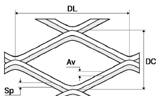
Maglia Romboidale
